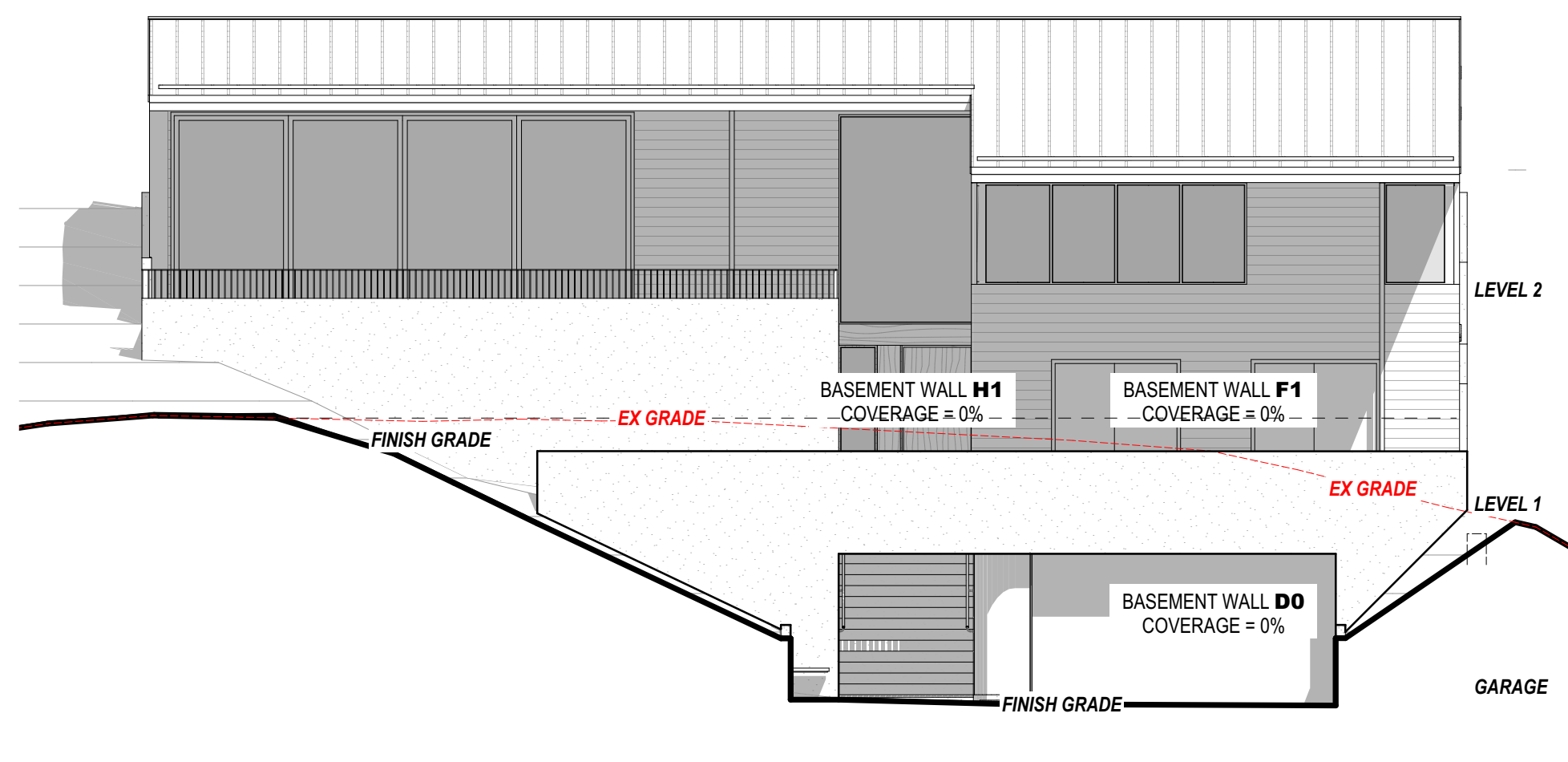
4 WEST ELEVATION SCALE: 1/8" = 1'-0"
