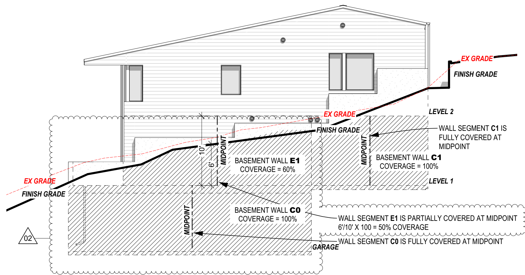
3 SOUTH ELEVATION SCALE: 1/8" = 1'-0"
